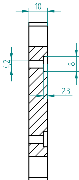
Schnitt A-A
